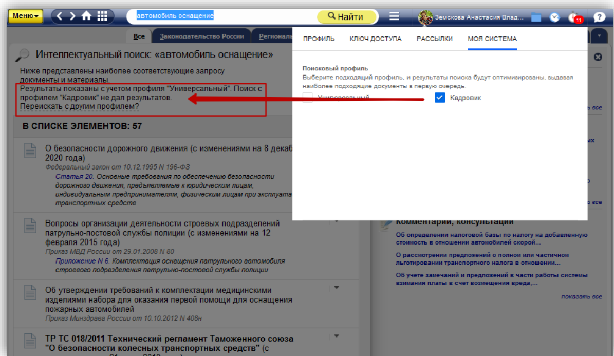
Рис.5 Обработка запроса, если поиск по профилю не даёт результата
