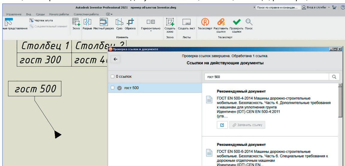
Рис. 36. Работа со ссылками в Inventor
